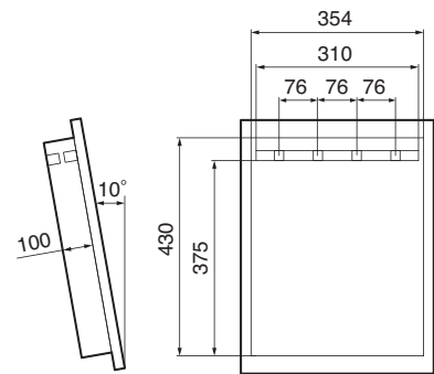
チャンバー寸法図(mm)
